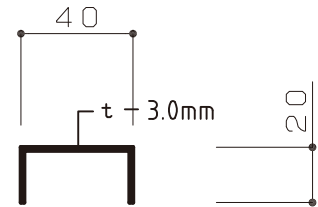
アルミチャンネル （市販品）
