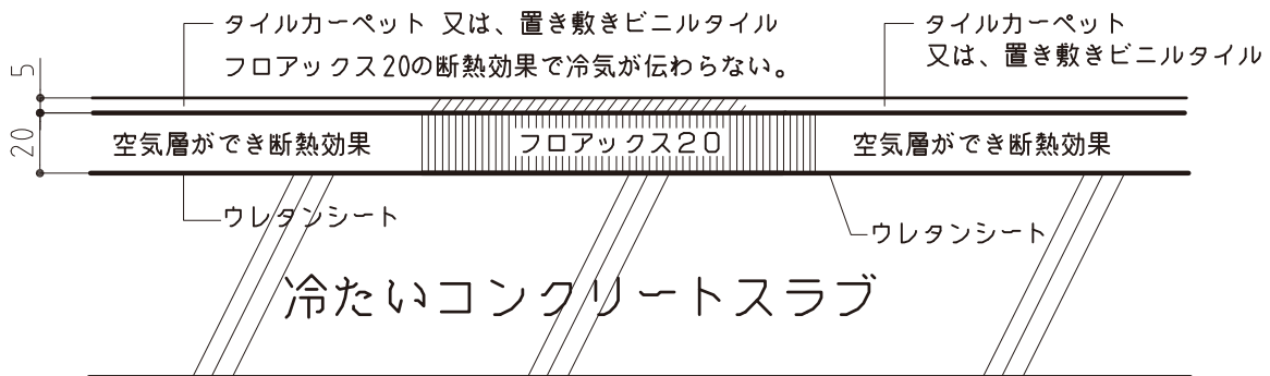
床断面図
