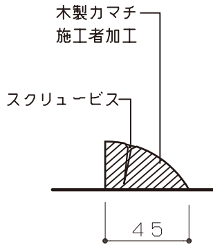
木製カマチ （施工者加工）
